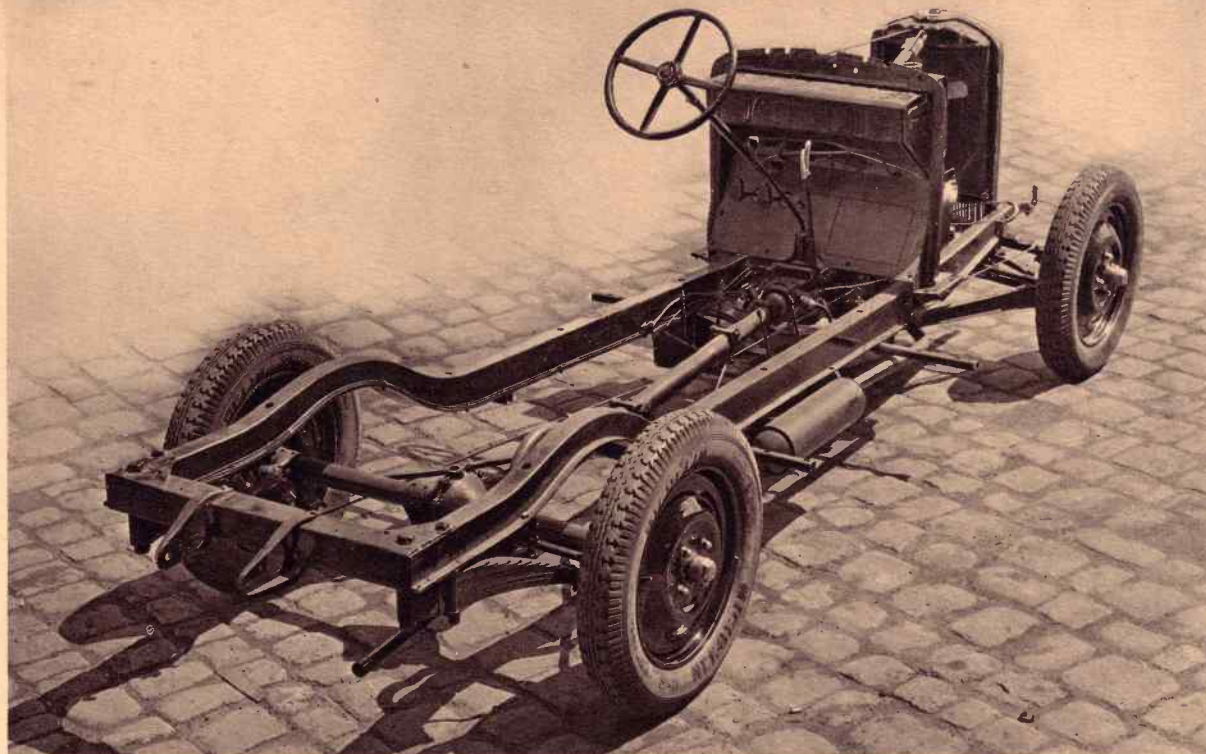
LE CHASSIS 301 "BLOCTUBE" A ROUES AVANT INDÉPENDANTES
