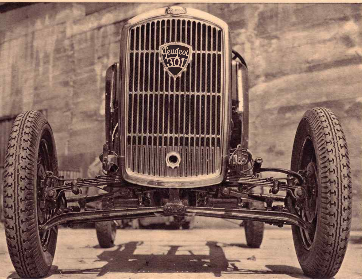
LE CHASSIS 301 "BLOCTUBE" A ROUES AVANT INDÉPENDANTES
