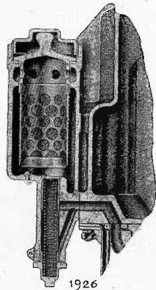
Fig. 21. Détail du filtre à huile démontable.
