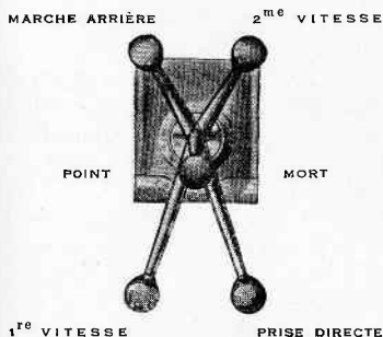
Fig. 33. - Schéma des positions du levier des vitesses sur les boîtes silencieuses et synchronisées (disposition standard).
