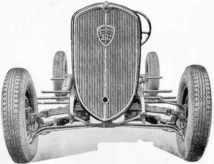
Fig. 1 Vue de face du châssis.
