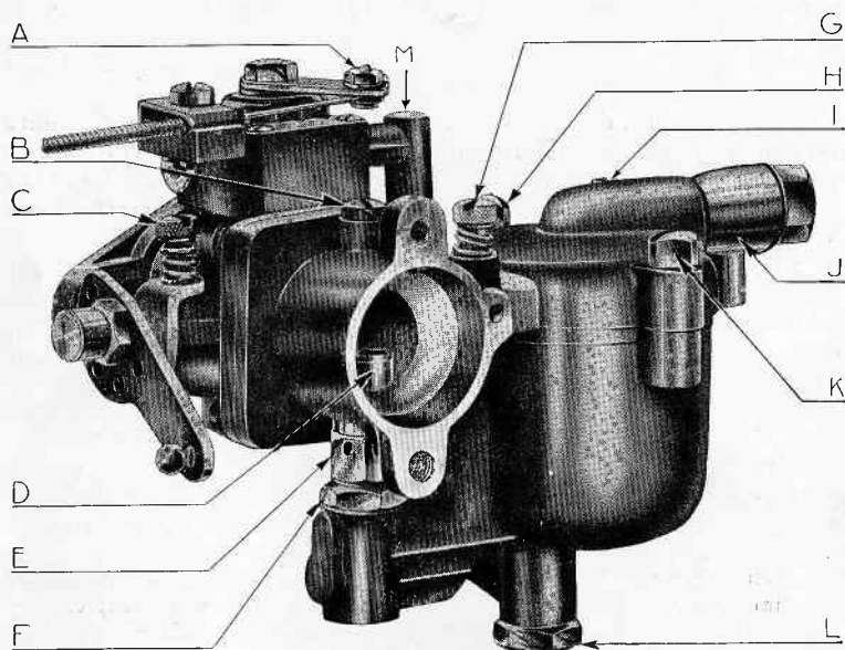
Fig. 13. — Carburateur.
