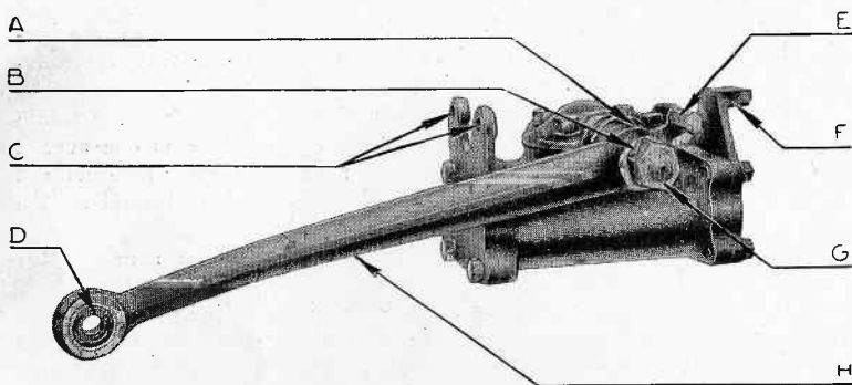
Fig. 8. — Amortisseur hydraulique.
