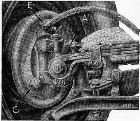
Fig 18. — Réglage des freins avant.
