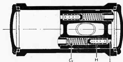
Fig. 10. — Coupe schématique montrant le fonctionnement des amortisseurs.
