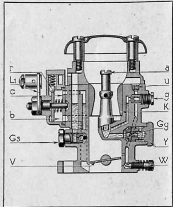
Fig. 11. — [Coupe longitudinale
