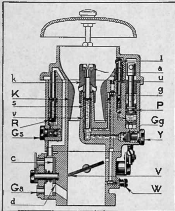
Fig. 19. — Coupe
