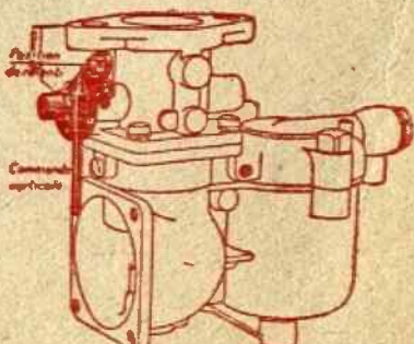
VBFG Commande verticale
