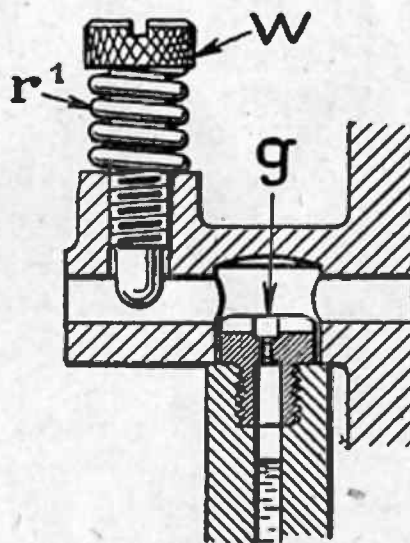
Fig. 9. — Carburateur FH à starter. Coupe par la vis de réglage d'air du ralenti.
